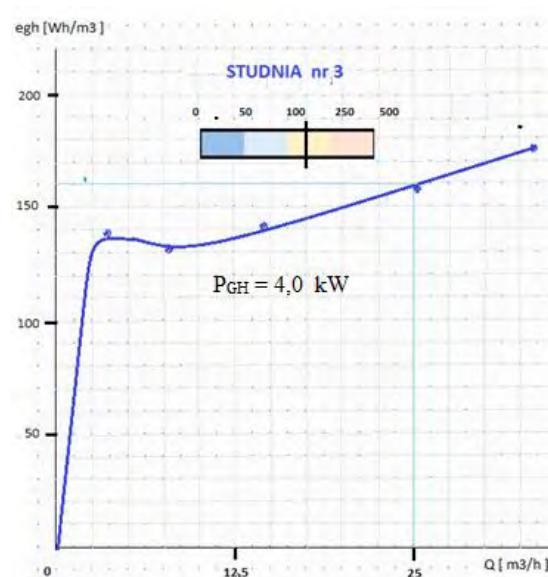
Ryc. 6. Zmienność wskaźnika dla przykładowej studni nr 3, która już po uruchomieniu osiąga e_{GH} > 100 \text{ Wh/m}^3
