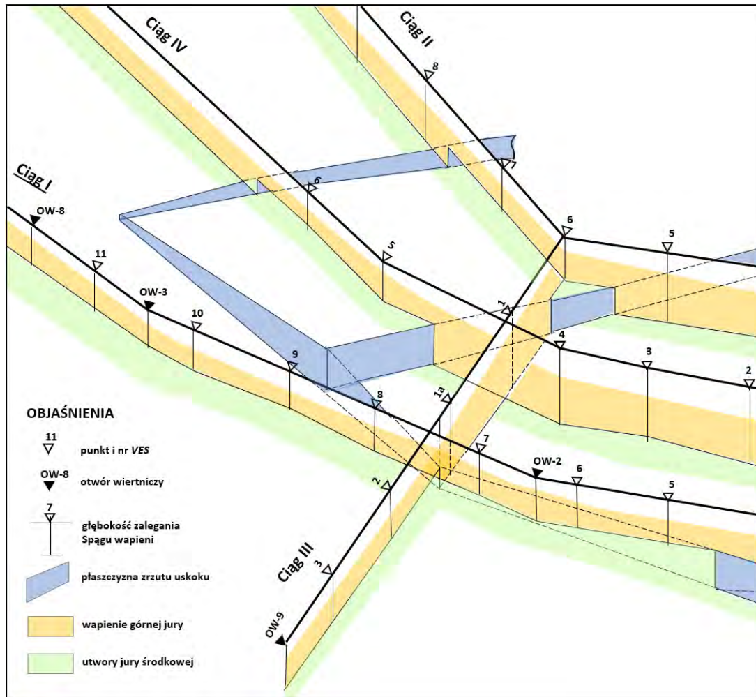
Ryc. 6. Archiwalne przestrzenne zestawienie przekrojów geoelektrycznych opartych o wyniki pionowych sondowań elektrooporowych w rejonie Łobodna
