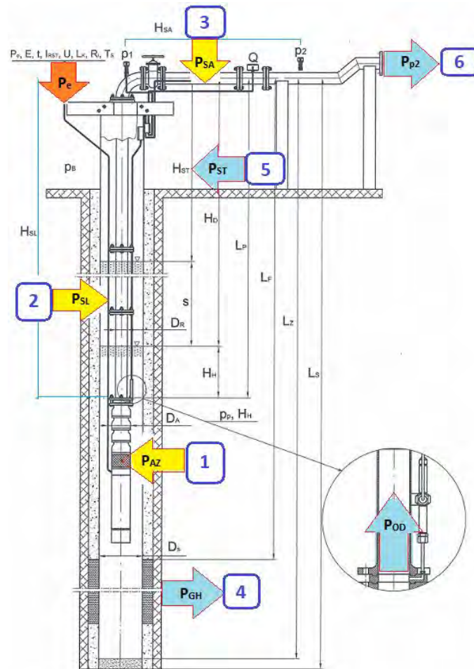
Ryc. 3. Schemat miejsc rozpraszania mocy pracującego układu pompowego studni głębinowej
