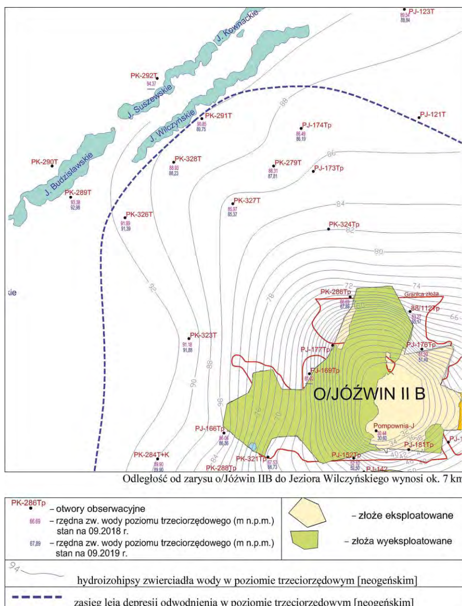
Ryc. 3. Sieć otworów obserwacyjnych (piezometrów) w rejonie jezior Powidzkiego Parku Krajobrazowego (Budzisławskie, Suszewskie, Wilczyńskie) oraz w otoczeniu O/Józwin IIB z postacią leja depresji w 2019 r.
