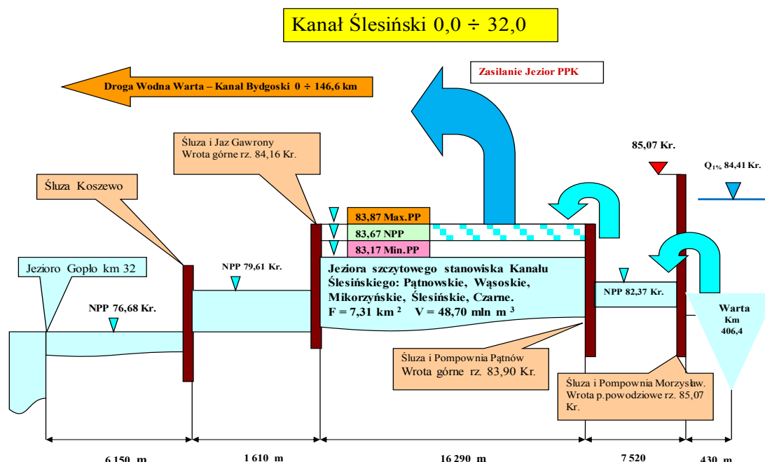
Ryc. 5. Poglądowy schemat szczytowego stanowiska Kanału Ślesińskiego jako miejsca poboru wody powierzchniowej do poprawy zasilania jezior PPK poprzez napełnianie końcowych zbiorników wodnych po odkrywkach PAK KWB Konin – schemat na ryc. 6
