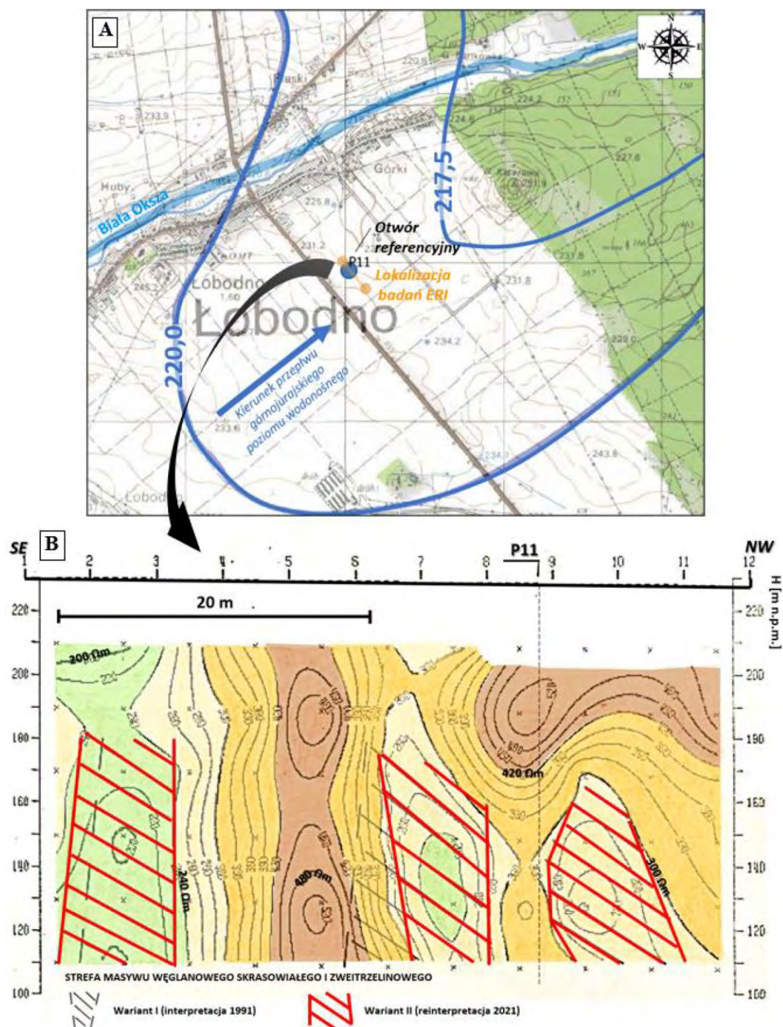
Ryc. 1. Mapa lokalizacyjna na tle topografii i kierunku przepływu górnajurajskich wód podziemnych (rozkład hydroizohips na podstawie Zdechlik i in. 2013, A), wybrany przekrój geoelektryczny (zmodyfikowane za Szymanko i Żyliński 1991, B)
