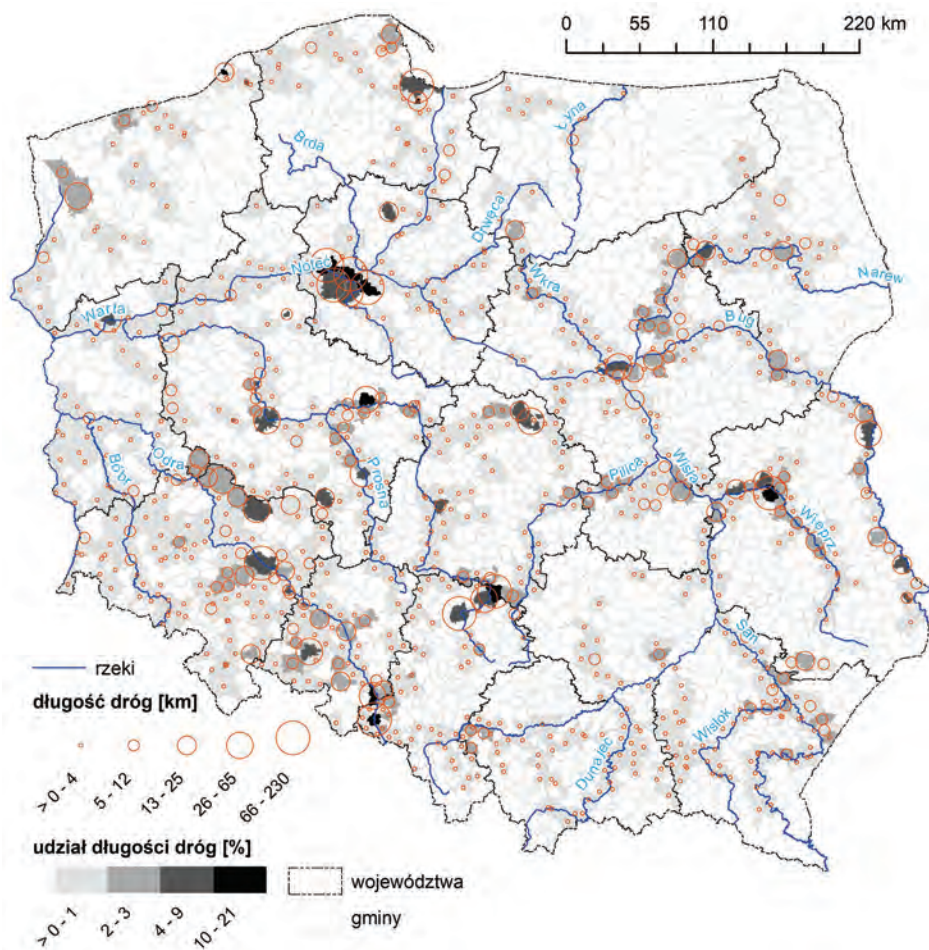
Ryc. 4.12. Długość „odciętych” odcinków dróg oraz ich udział w całkowitej długości dróg w gminach w przypadku wystąpienia powodzi o prawdopodobieństwie 10% w Polsce w 2019 r.
