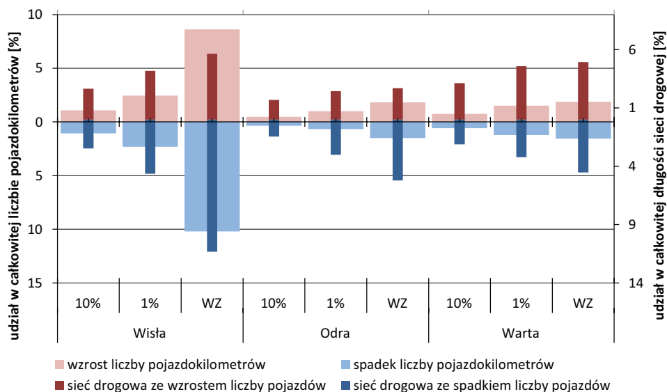
Ryc. 7.30. Względne zmiany liczby pojazdokilometrów towarzyszące podróżom służbowym w następstwie wystąpienia powodzi na głównych rzekach w określonym scenariuszu w Polsce w 2019 r.
