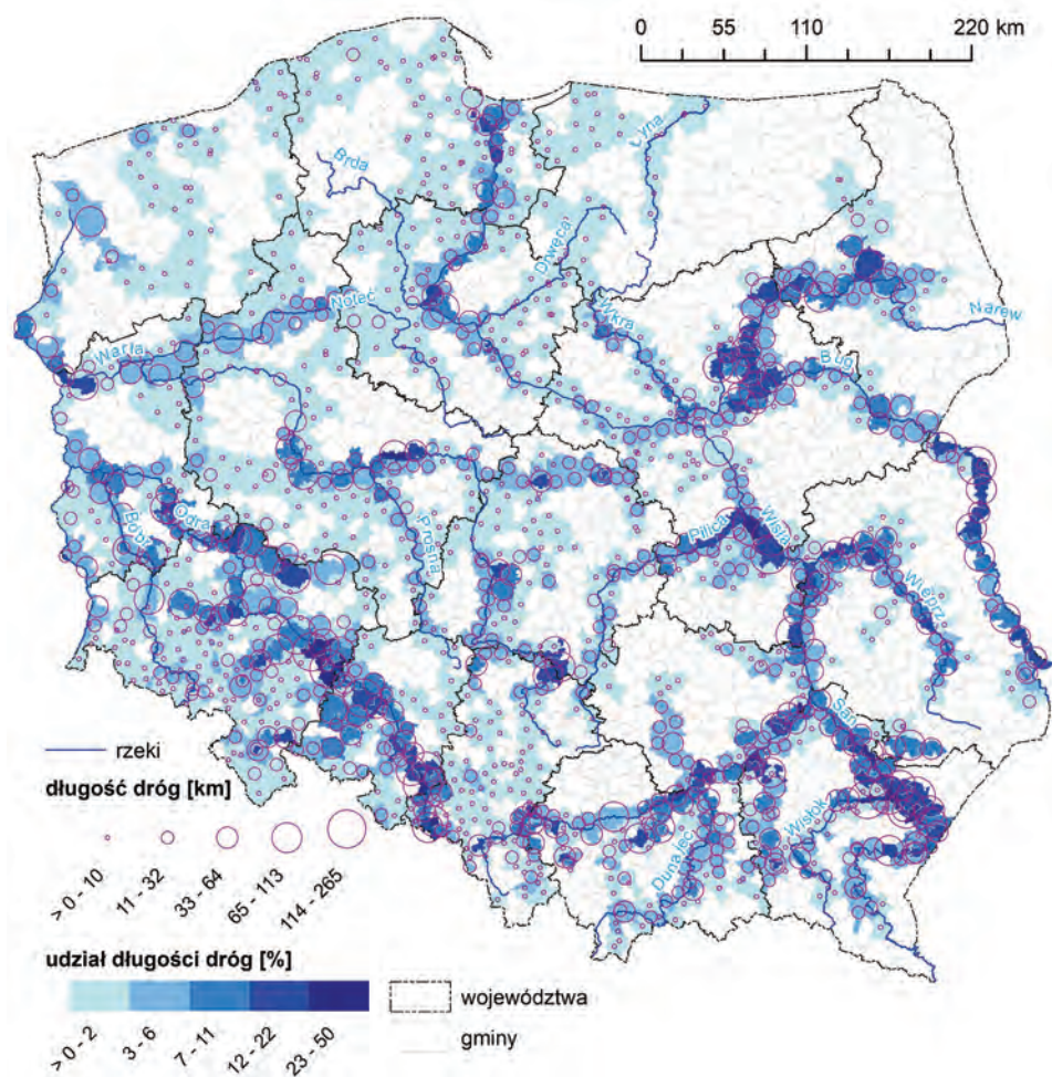
Ryc. 4.8. Długość zalanych odcinków dróg oraz ich udział w całkowitej długości dróg w gminach w przypadku wystąpienia powodzi od rzeki o prawdopodobieństwie 1% w Polsce w 2019 r.
