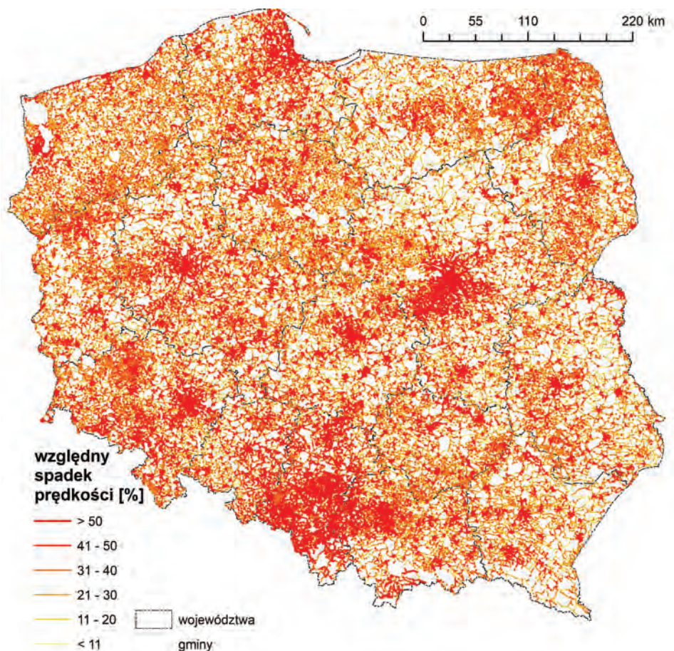
Ryc. 5.5. Względne spadki prędkości przejazdu odcinka sieci wynikające z zastosowania modelu prędkości ruchu względem prędkości kodeksowych w Polsce w 2019 r.
