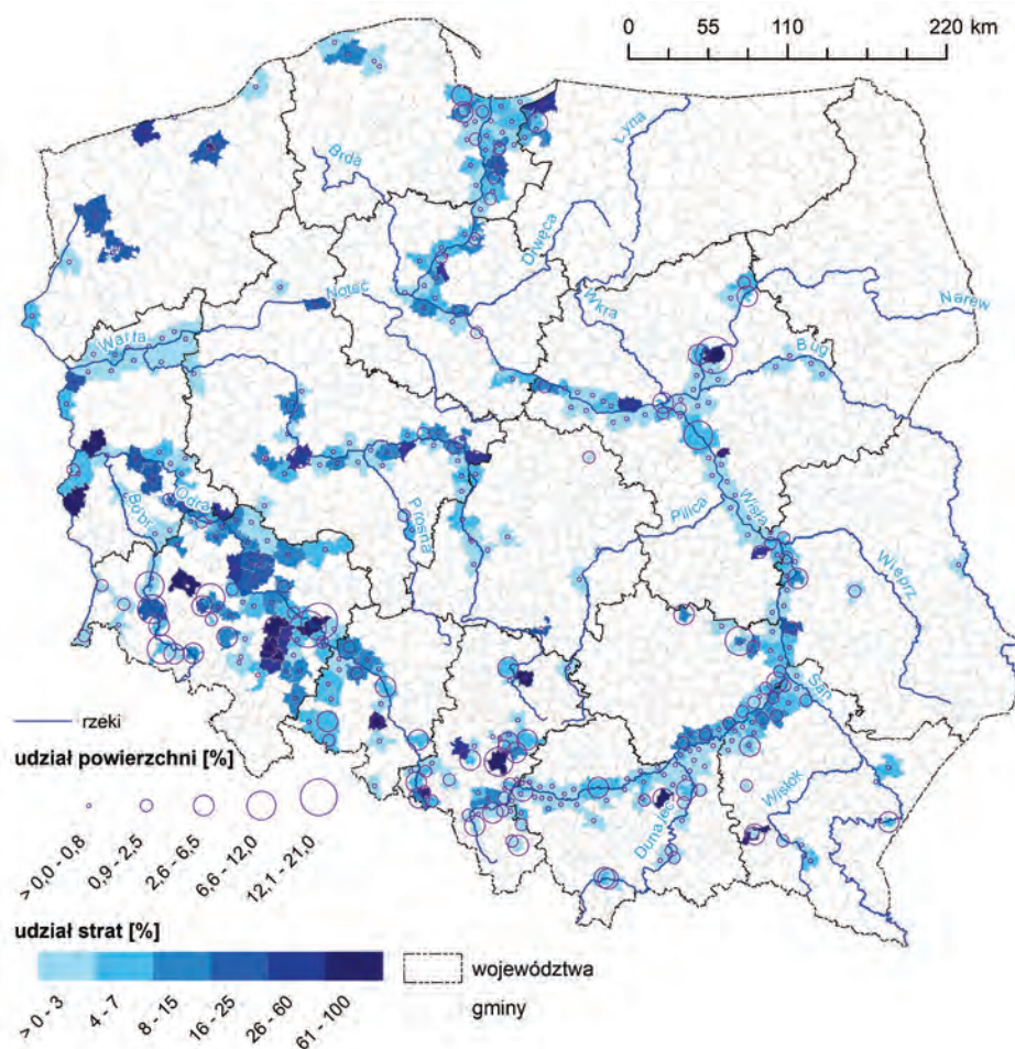
Ryc. 3.23. Udział powierzchni oraz potencjalnych strat wynikających z zalania terenów komunikacyjnych w ogóle powierzchni terenów zagrożonych i potencjalnych strat w gminach na skutek wystąpienia powodzi w przypadku całkowitego zniszczenia obwałowania w Polsce w 2019 r.
