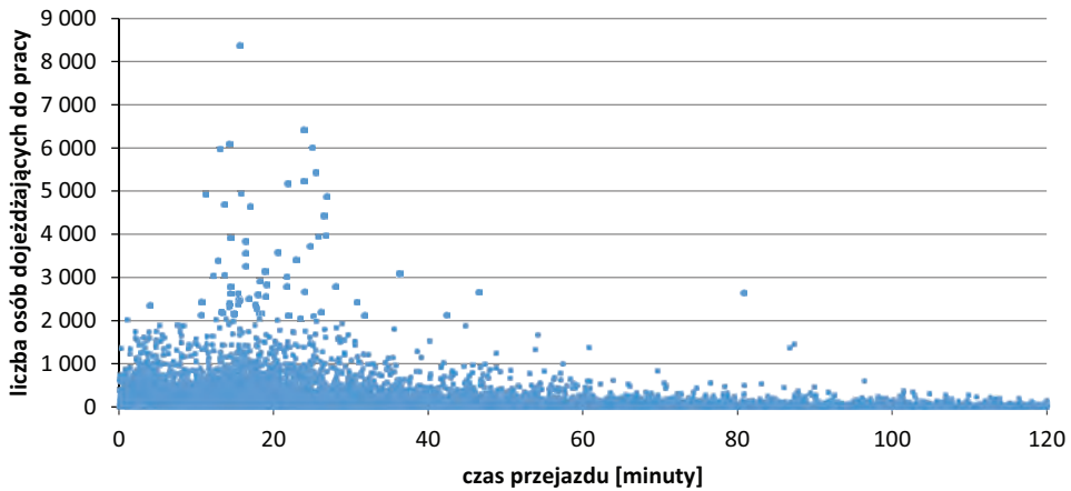
Ryc. 5.21. Liczba osób dojeżdżających do pracy w Polsce w 2016 r. w stosunku do długości trwania podróży realizowanej samochodem osobowym Źródło: opracowanie własne na podstawie danych GUS, 2019 r.
