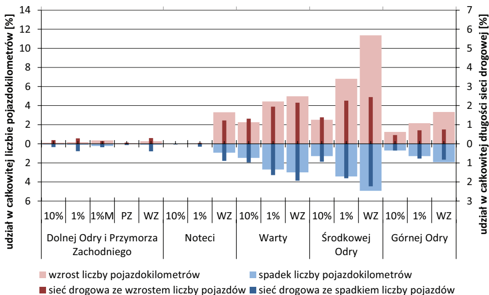
Ryc. 7.10. Względne zmiany liczby pojazdokilometrów towarzyszące dojazdom do pracy w następstwie wystąpienia powodzi w określonym scenariuszu na obszarze dorzecza Odry wg regionów wodnych w Polsce w 2019 r.
