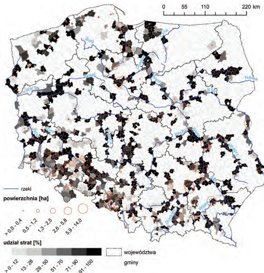
Ryc. 3.24. Powierzchnia oraz udział potencjalnych strat związanych z zalaniem terenów pod drogami kołowymi w ogóle zagrożonych terenów komunikacyjnych w przypadku wystąpienia powodzi o prawdopodobieństwie 10% w Polsce w 2019 r.
