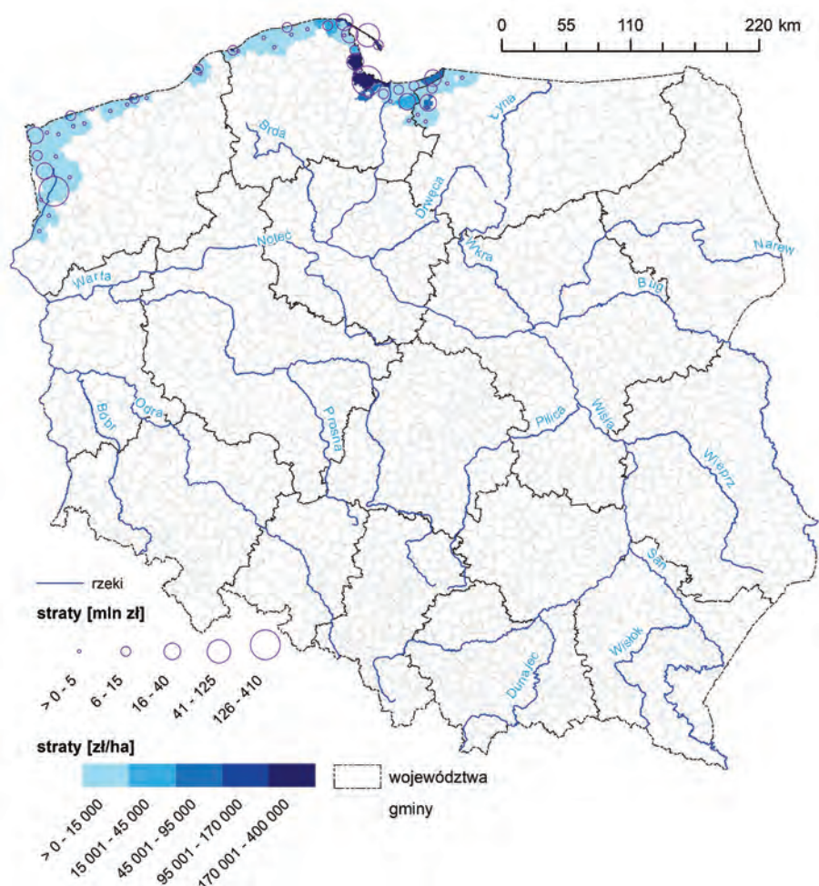
Ryc. 3.16. Przypadające na hektar terenów zagrożonych oraz całkowite wielkości potencjalnych strat materialnych związanych z wystąpieniem powodzi od morza o prawdopodobieństwie 1% w Polsce w 2019 r.
