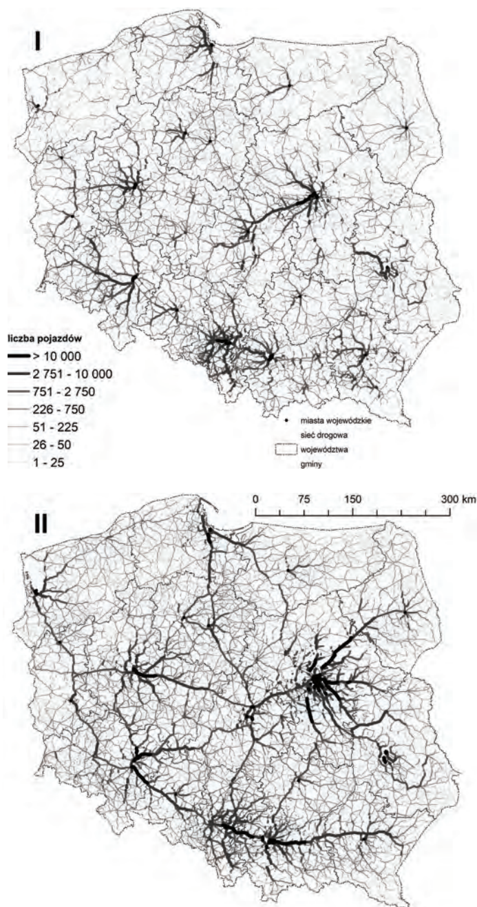
Ryc. 5.24. Obciążenie sieci drogowej w wyniku realizacji dojazdów do pracy (I) oraz podróży służbowych (II) w Polsce
