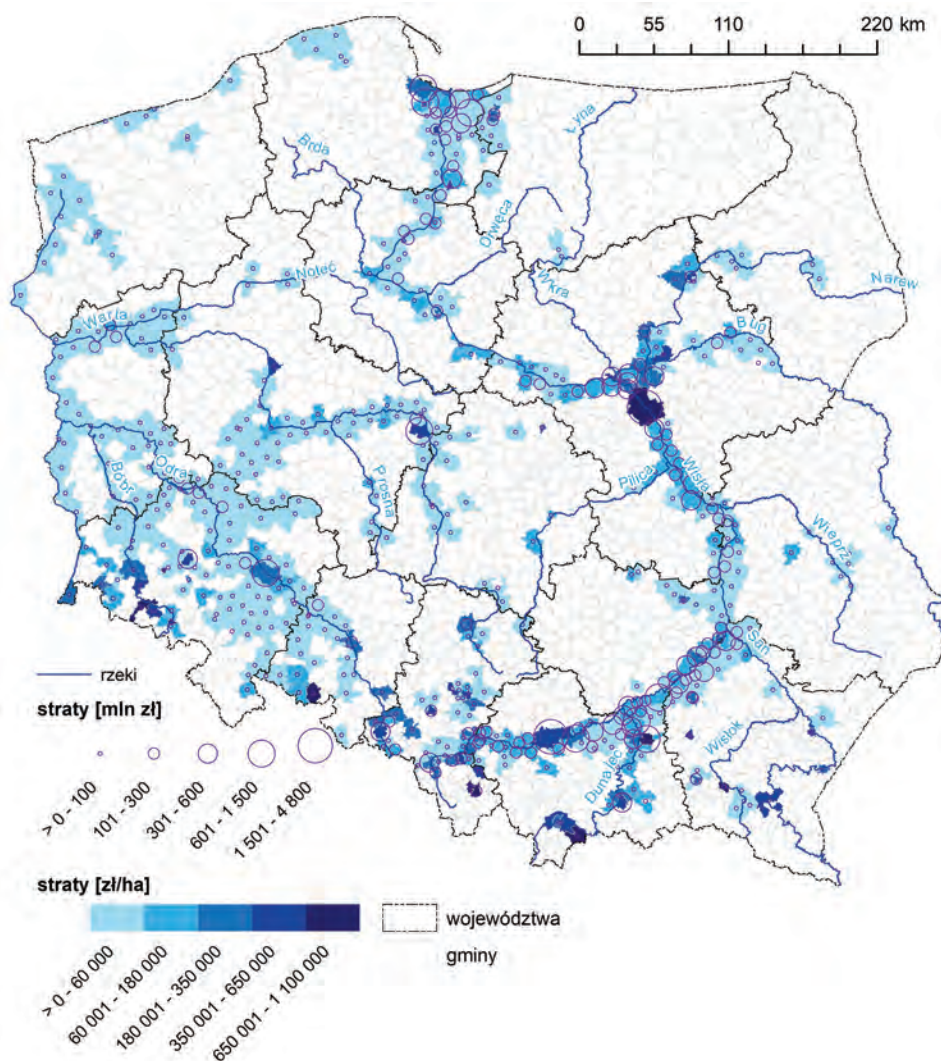
Ryc. 3.18. Przypadające na hektar terenów zagrożonych oraz całkowite wysokości potencjalnych strat materialnych związanych z wystąpieniem powodzi w przypadku całkowitego zniszczenia obwałowania w Polsce w 2019 r.
