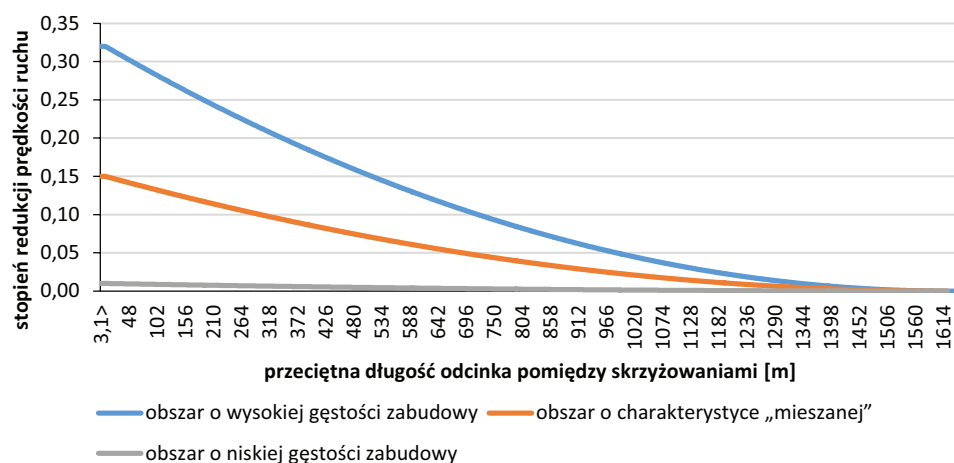
Ryc. 5.2. Redukcja prędkości spowodowana zagęszczeniem skrzyżowań dla dróg krajowych
