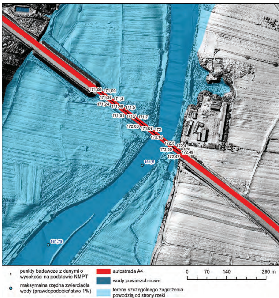
Ryc. 4.5. Przykład zestawienia danych NMPT i maksymalnej rzędnej zwierciadła wody (most na Odrze w ciągu autostrady A4) w 2019 r.
