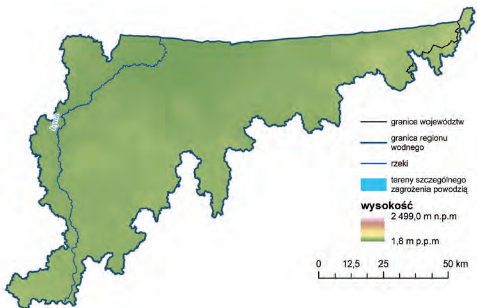
Ryc. 3.7. Tereny zagrożone powodzią na tle ukształtowania powierzchni terenu na obszarze dorzecza Pregoly w 2019 r.
